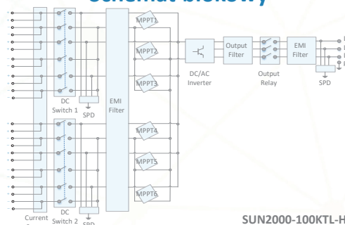
Schemat blokowy
