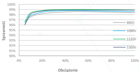
Krzywa sprawności
