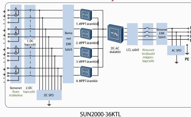
Áramköri rajz
