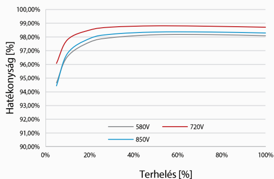
Hatásfok görbe
